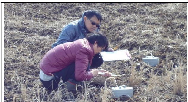
千葉県横芝における圃場からのガス採取 Gas sampling at field experiment in Yokoshiba Chiba Prefecture
